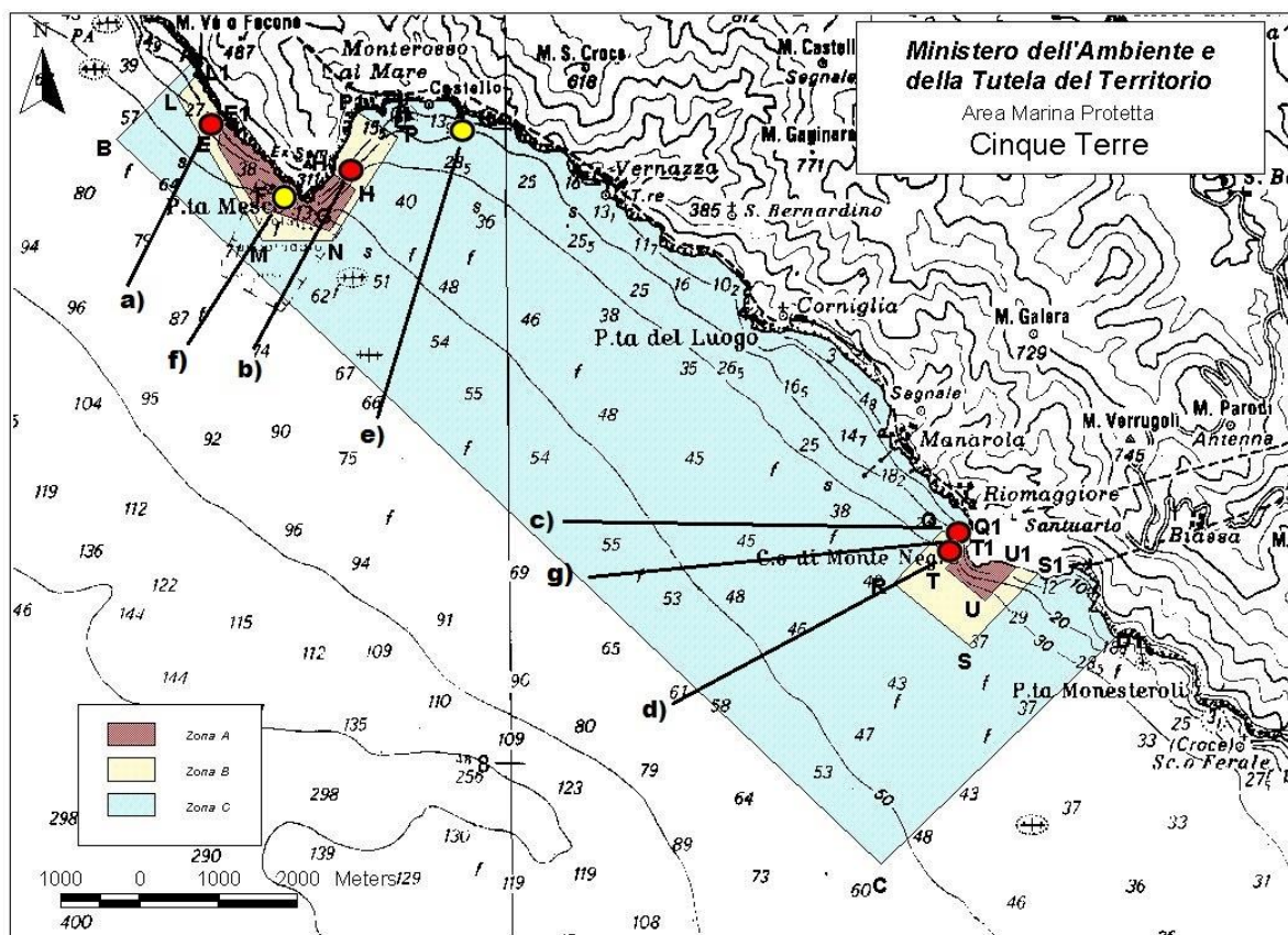
Figura 7: Gavitielli singoli riservati alle unità navali in appoggio alle visite guidate subacquee
